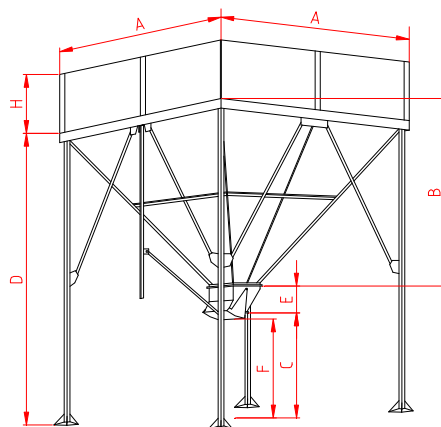
TREMIE AVEC CASQUE DE VIDAGE MANUEL
